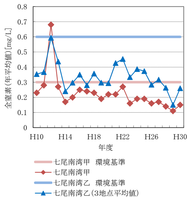
■ 図 3-5 七尾南湾 全窒素濃度経年変化
