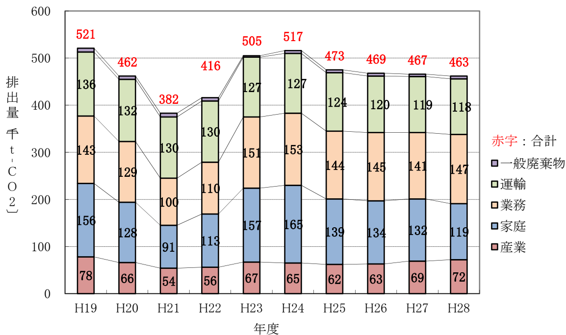
■図 8-2 七尾市の二酸化炭素排出量
