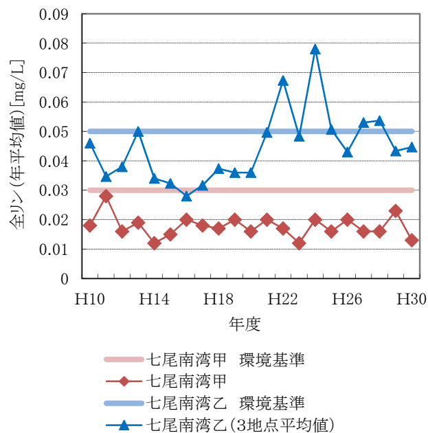
■ 図 3-6 七尾南湾 全リン濃度経年変化
