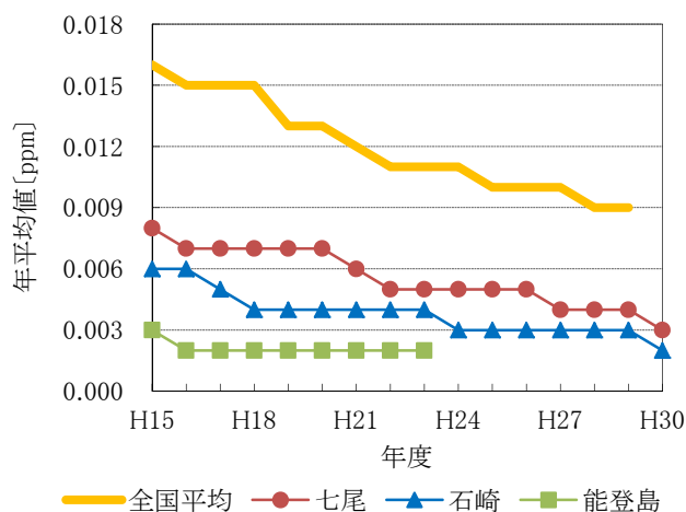
■図 2-3 NO 2 年平均値の経年変化
