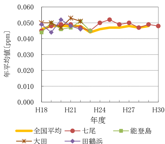
■図 2-5 Ox 昼間の日最高 1 時間値の 年平均値の経年変化
