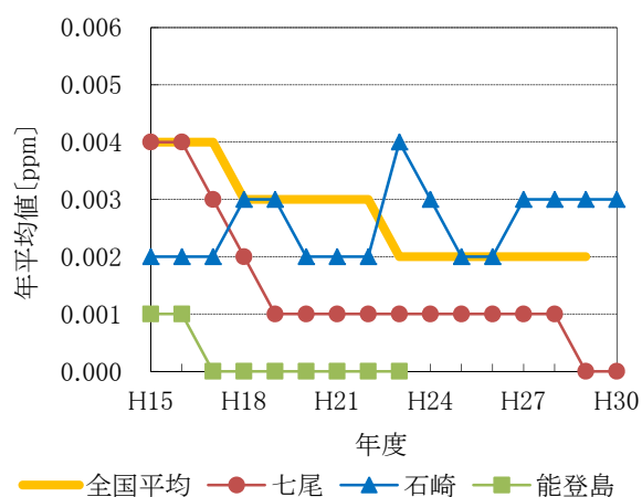
■図 2-2 SO 2 年平均値の経年変化
