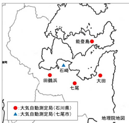
■図 2-1 大気測定局 位置図
