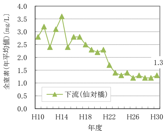
■図 3-8 御祓川 全窒素濃度経年変化
