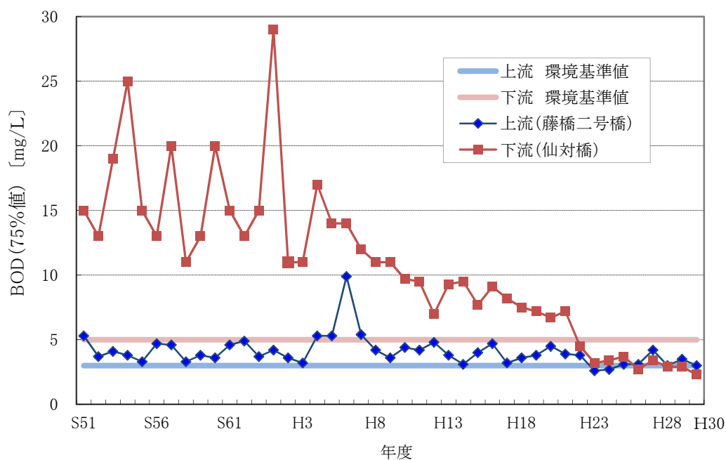
■図 3-7 御祓川 BOD 濃度経年変化
