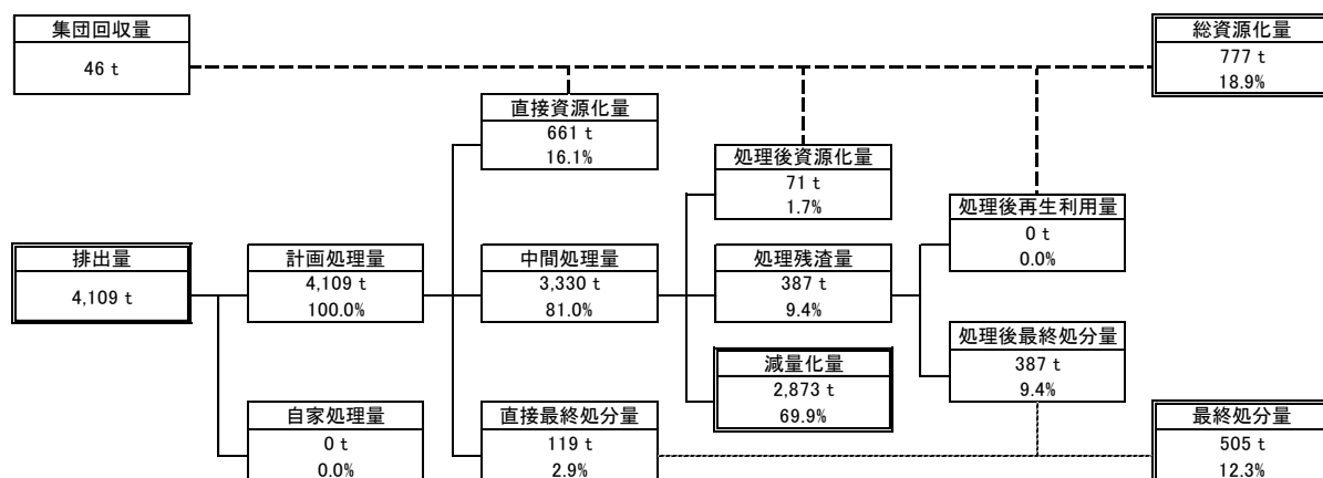
図8 【中能登町】目標達成時のごみ処理状況フロー（令和5年度）
