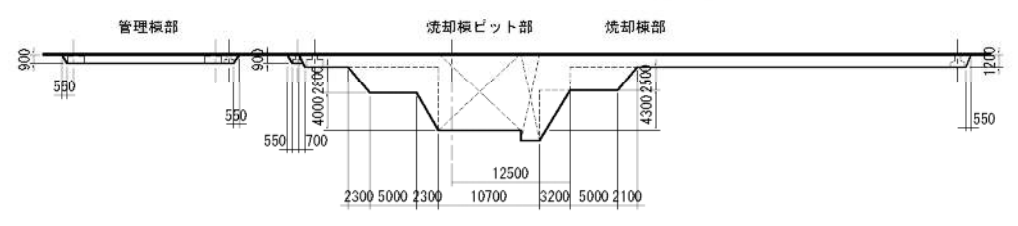
B-B断面図
