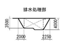
C-C断面図
